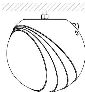
顶挂方式：使用M6螺杆和螺母 顶挂(螺杆和螺母，客户自备)
